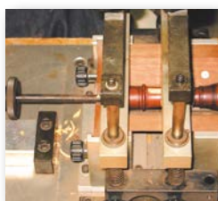
5 ウィンドウェイを削る 専用の工具でウィンドウェイを削ります。
