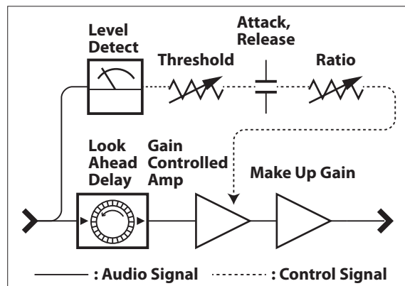
本機のコンプレッサーの構成
