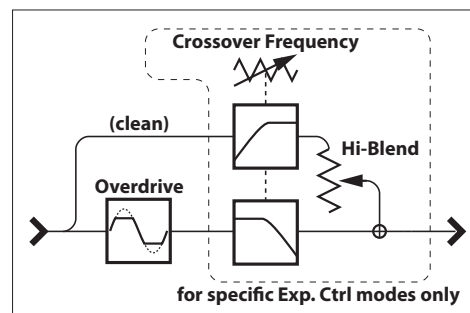
本機のオーバードライブの構成
