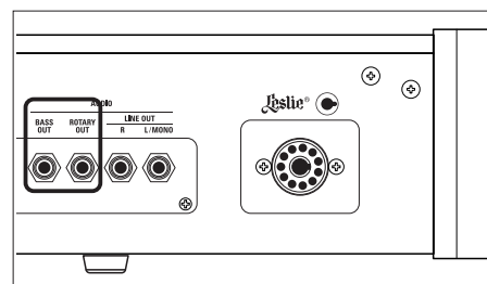
BASS OUTジャックとROTARY OUTジャック
