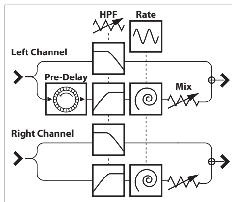
本機のコーラスの構成
