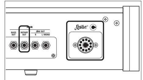
ROTARY OUTジャックとレズリー・ソケット
