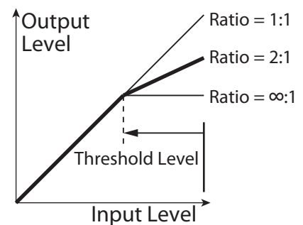
コンプレッサーの概念図
