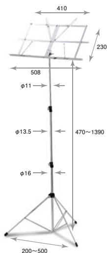
MS-400 単位 (mm)
