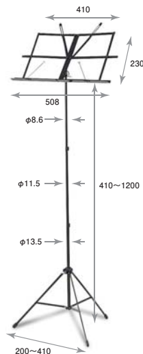
MS-300B 単位 (mm)
