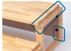
●ジョイントする場合
