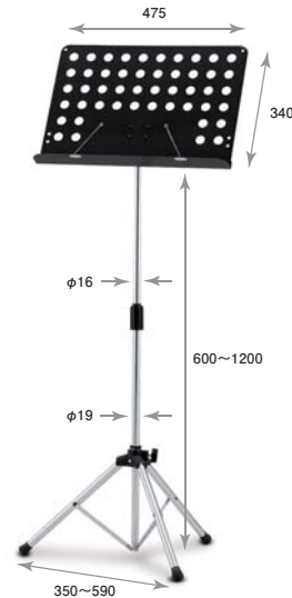
単位(mm)
