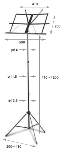
MS-300B 単位 (mm)
