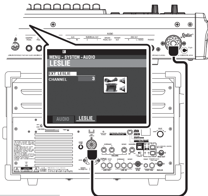
3チャンネル・タイプとの接続例
