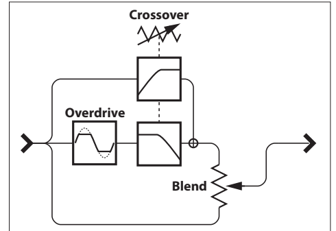
本機のオーバードライブの構成
