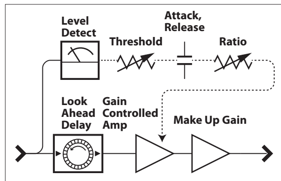
本機のコンプレッサーの構成
