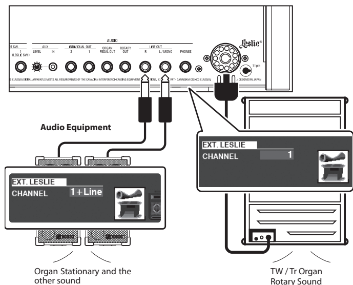
1チャンネル・タイプとの接続例
