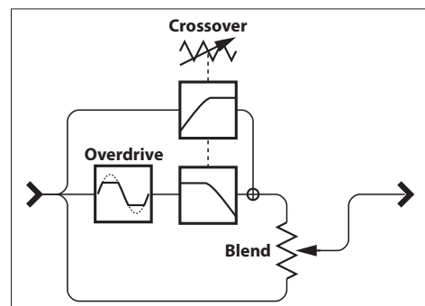
本機のオーバードライブの構成
