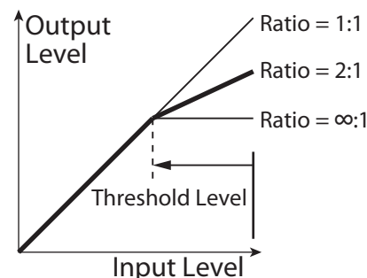
本機のコンプレッサーの構成
