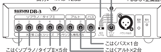
▽DB-3&lt;正面図&gt;
